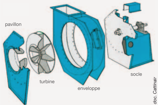
Fig. 7 Principe du ventilateur centrifuge
